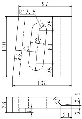
② 座 金 SS400
