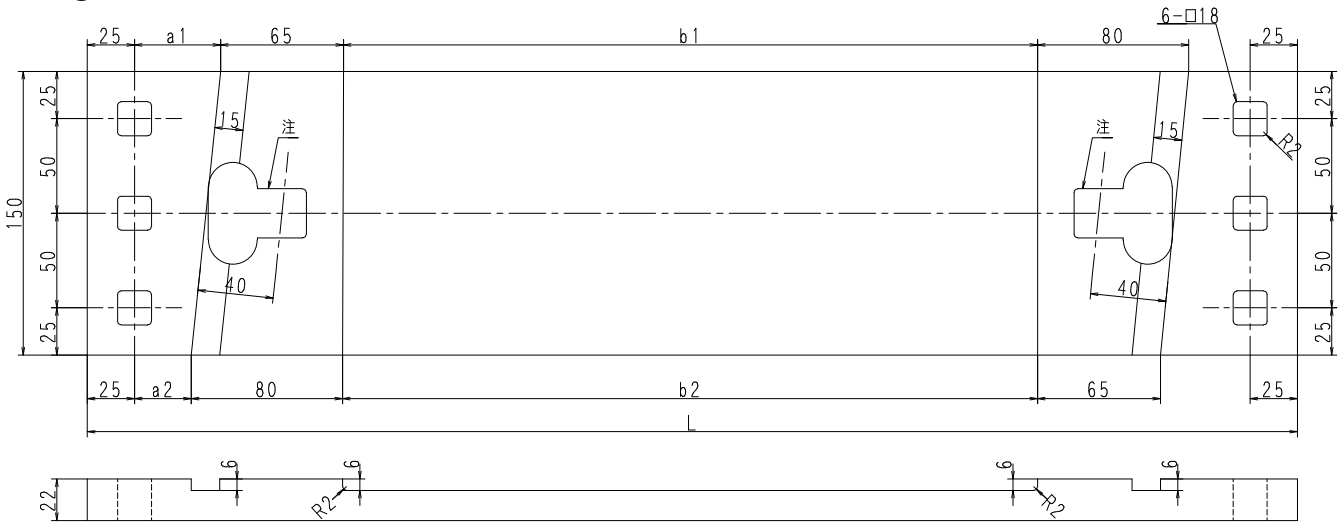
① タイプレート本体 SS400
